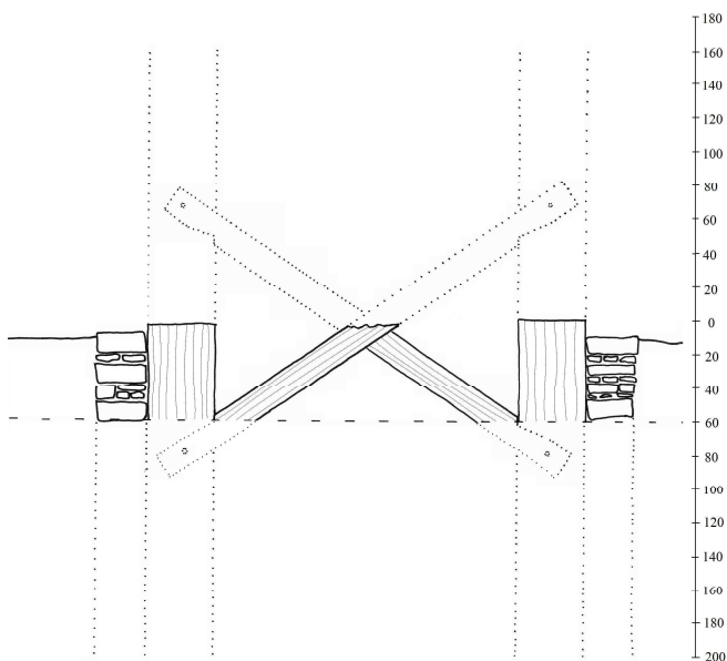
Rekonstrukce ondřejského kříže, plnou čarou odhalené konstrukce, tečkovaně doplněný rozsah.
